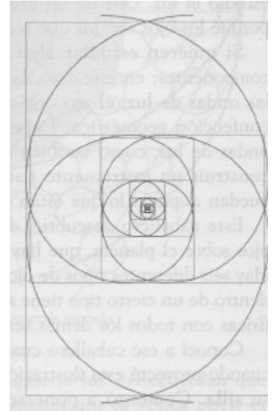
Fig. 12-22a: La geometría de la luz en espirales de proporción áurea.
