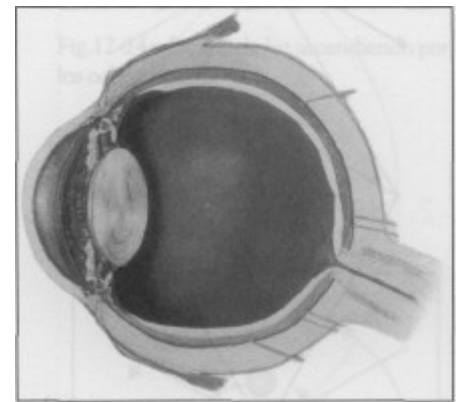
Fig. 12-19: El ojo humano.
